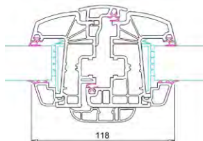
Battement central fenêtre (162 mm en porte-fenêtre serrure)
