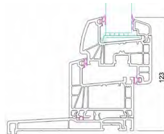
Pièce d'appui
