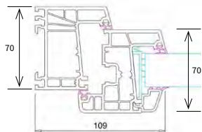
Montant latéral
