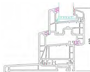
Pièce d'appui
