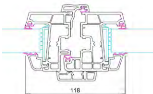
Battement central fenêtre (162 mm en porte-fenêtre serrure)
