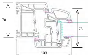
Montant latéral
